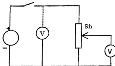
Aufbau Potentiometer
